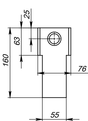
Поз.5 (Пластина)
