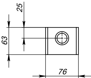
Поз.4 (Пластина)
